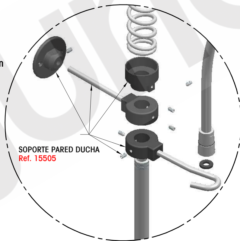
DETALLE A
