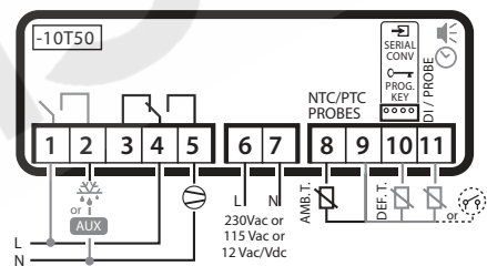
PJEZ(S, X)*
