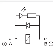
C: Variantes 6, 7, 74 LED + diodo (DC, positivo en A/A1)
