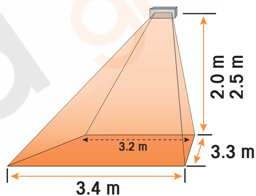
MONTAJE DE PARED A 45 GRADOS
